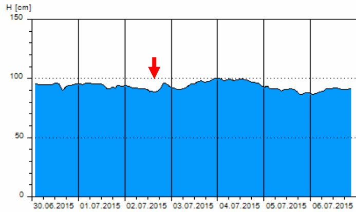
Stanice: LG Plzeň - Bílá Hora Tok: Berounka
