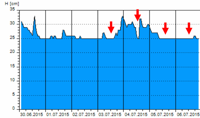
Stanice: LG Liblín Tok: Berounka
